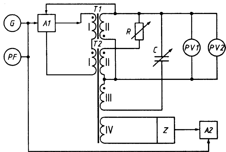
Рисунок 1 — Схема для измерений мостовым методом
